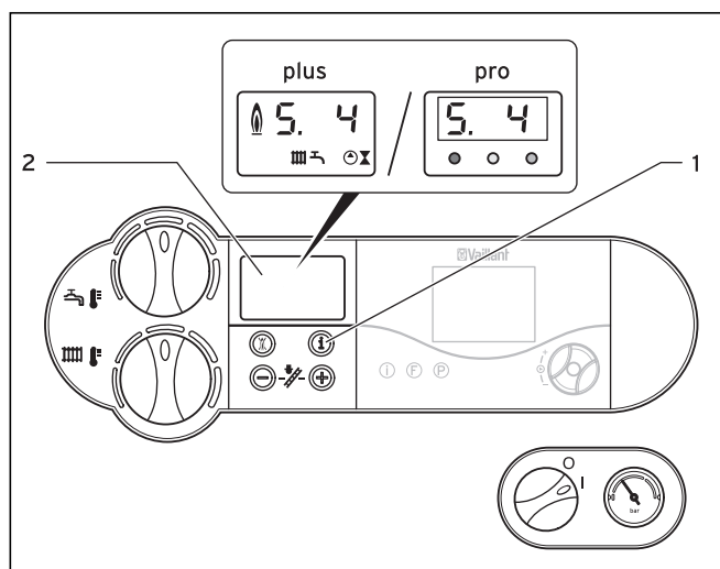
Fig. 4.17 Indicateurs d'état
