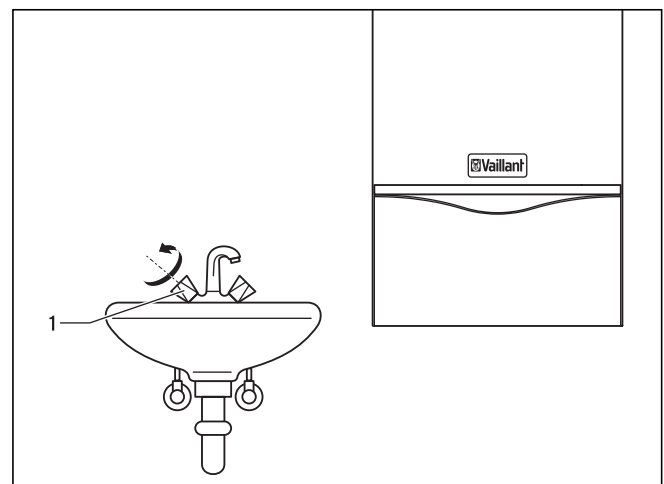
Fig. 4.10 Puisage d'eau chaude
