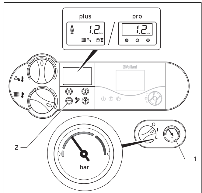
Fig. 4.5 Contrôle de la pression de remplissage de l'installation de chauffage
